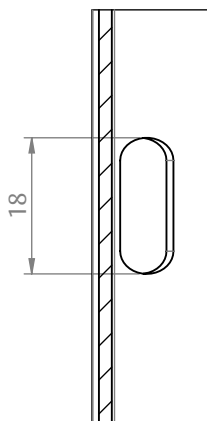
SEÇÃO A-A ESCALA 1 : 1
