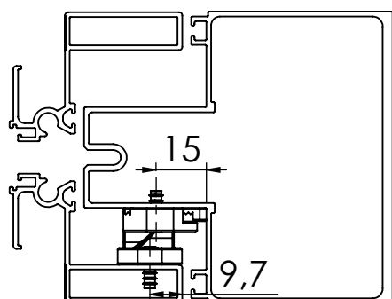
PERFIL - WALL FRAME
