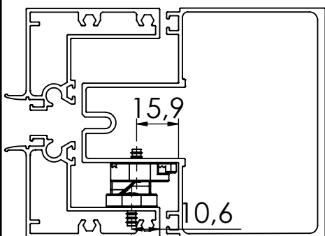
CDA - DA VINCI
