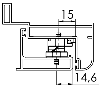
KAWNEER - CITTA DUE
