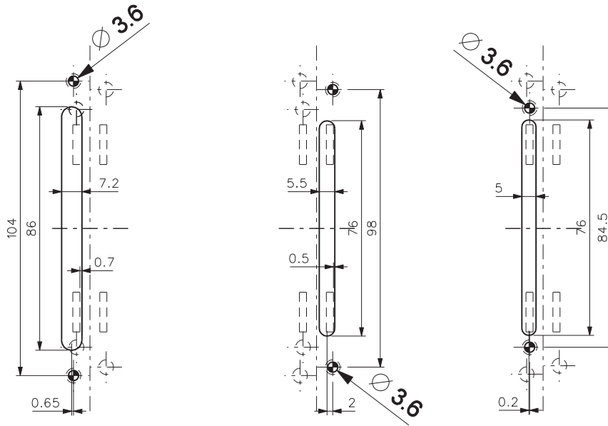
DETALHE DE USINAGEM PARA FIXAÇÃO DA CREMONA
