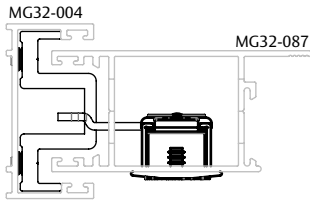
MEGA 32 (ASA ALUMÍNIO)
