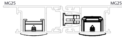
MEGA 25 (ASA ALUMÍNIO)
