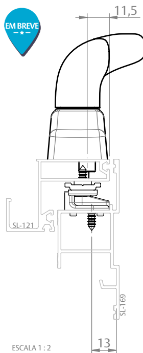
FACHADA SOLUTA (HYDRO)
