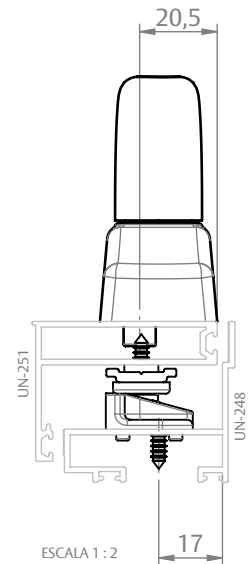
FACHADA UNIT (HYDRO)
