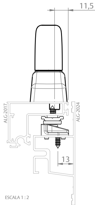
FACHADA SHADOW (CDA)
