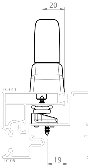
FACHADA CITTA (HYDRO)
