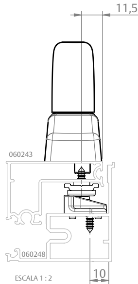
FACHADA ELEGANCE (HYDRO)
