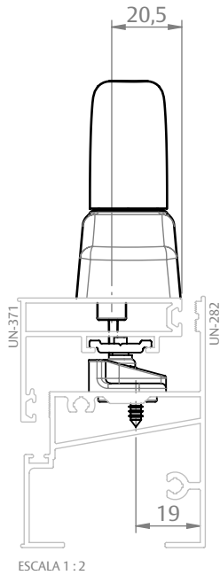
FACHADA UNIT (HYDRO)
