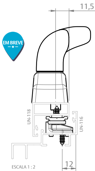
FACHADA UNIT (HYDRO)
