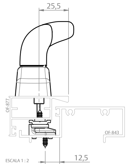
FACHADA OFFSET (BELMETAL)
