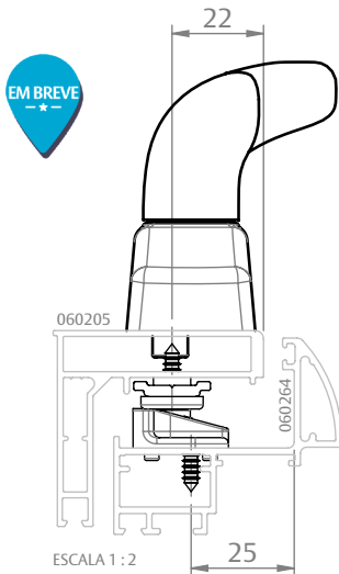
FACHADA ELEGANCE (HYDRO)
