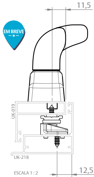
FACHADA UNIK (OLGA COLOR)
