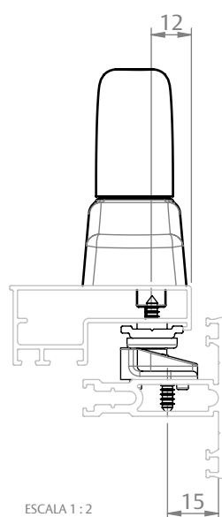
FACHADA STICK (SELTA)
