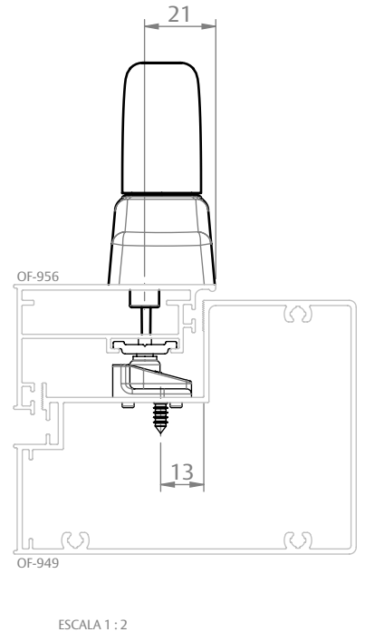
FACHADA OFFSET (BELMETAL)
