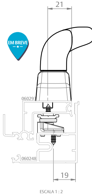
FACHADA PELE VIDRO (HYDRO)
