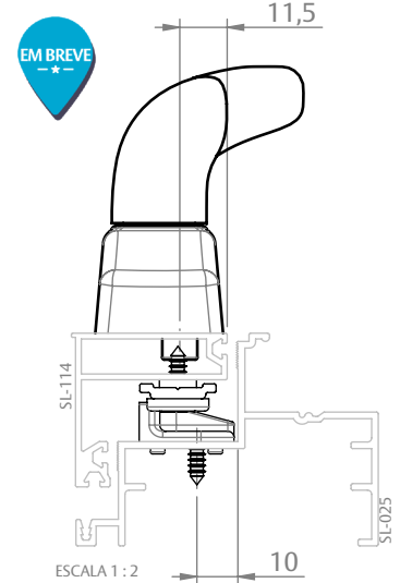
FACHADA SOLUTA (HYDRO)
