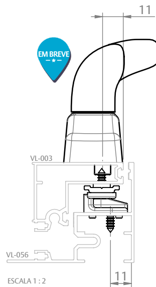
FACHADA CITTA DUE (HYDRO)
