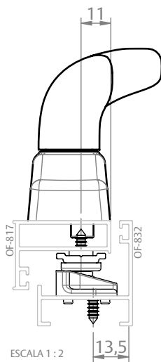
FACHADA OFFSET (BELMETAL)
