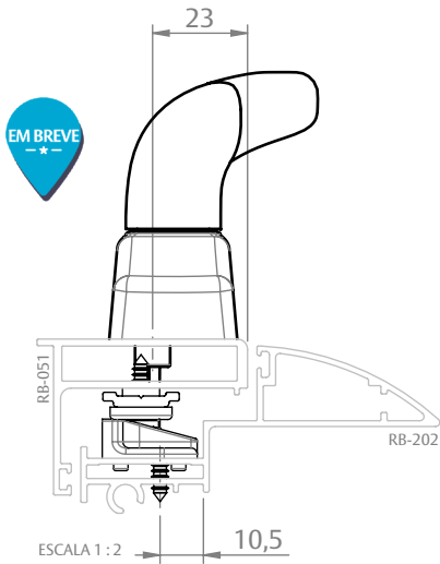
FACHADA REMBRANDT (CDA)
