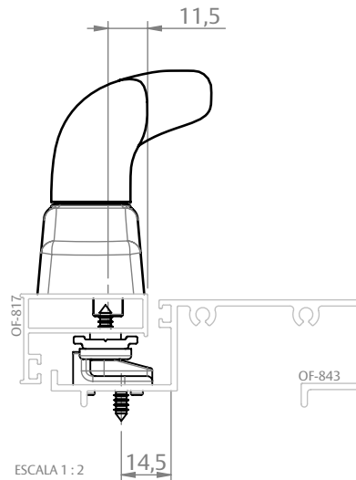
FACHADA OFFSET (BELMETAL)
