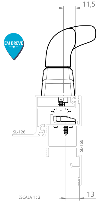
FACHADA SOLUTA (HYDRO)
