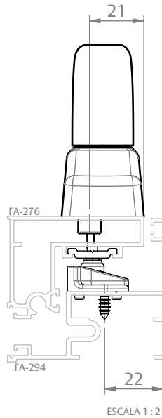
FACHADA ATLANTA (BELMETAL)
