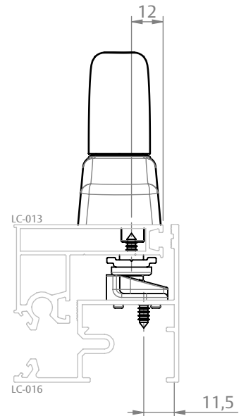
FACHADA CITTA (HYDRO)
