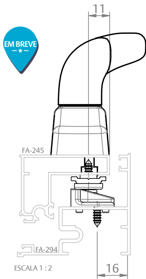
FACHADA ATLANTA (BELMETAL)
