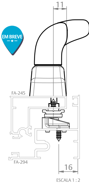
FACHADA ATLANTA (BELMETAL)
