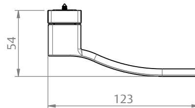
ESCALA 1 : 3
