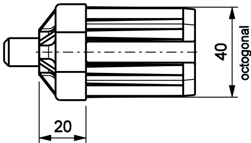
Ponteira OCT40
