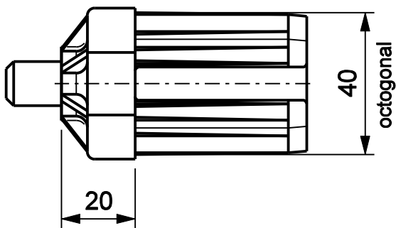
Ponteira OCT40
