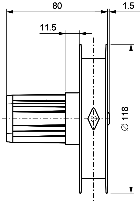
Polia
