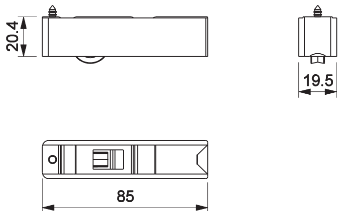
ROLDANA COM REGULAGEM E ROLAMENTO escala 1:2
